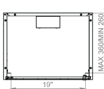
SECTION A-A SCALE 1 : 10
