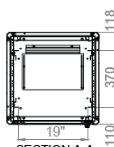
SECTION A-A SCALE 1 : 15
