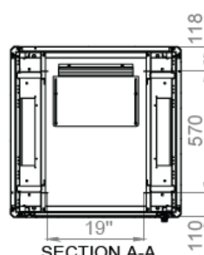
SECTION A-A SCALE 1 : 16
