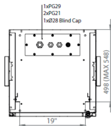
SECTION A-A SCALE 1 : 12
