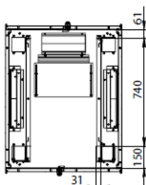
KESIT A-A
